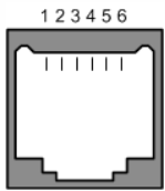
Connecteur RJ12
