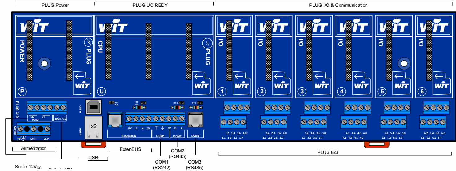
Exemple de localisation des raccordements du Connect-DIN UC REDY P6
