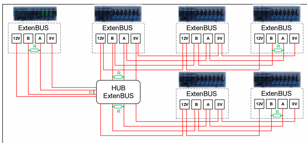
c) Topologie étoile et linéaire (avec HUB ExtenBUS)
