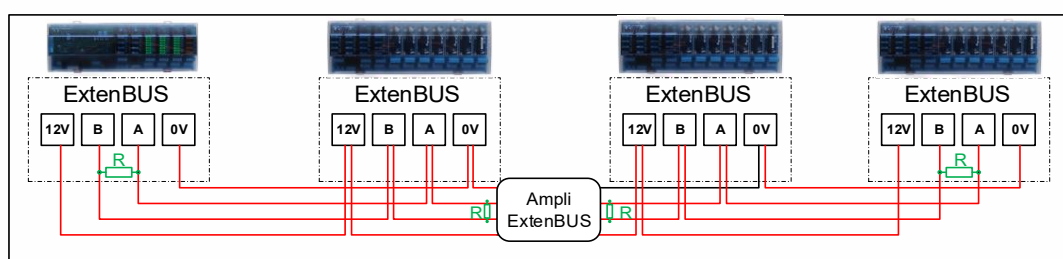
c) Topologie étoile et linéaire (avec HUB ExtenBUS)
