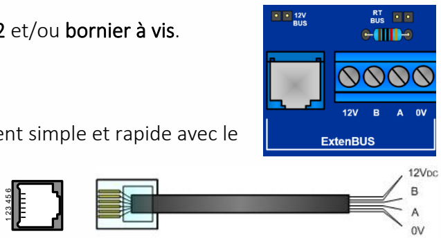
Cordon ExtenBUS
